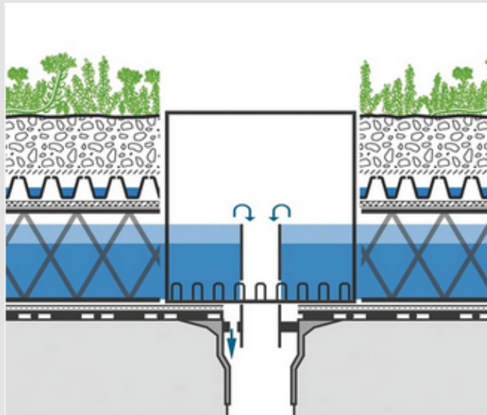
Retentionsgründach
