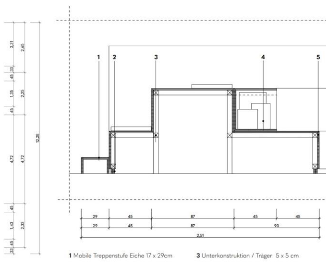
Detail Tribühne M 1:10
