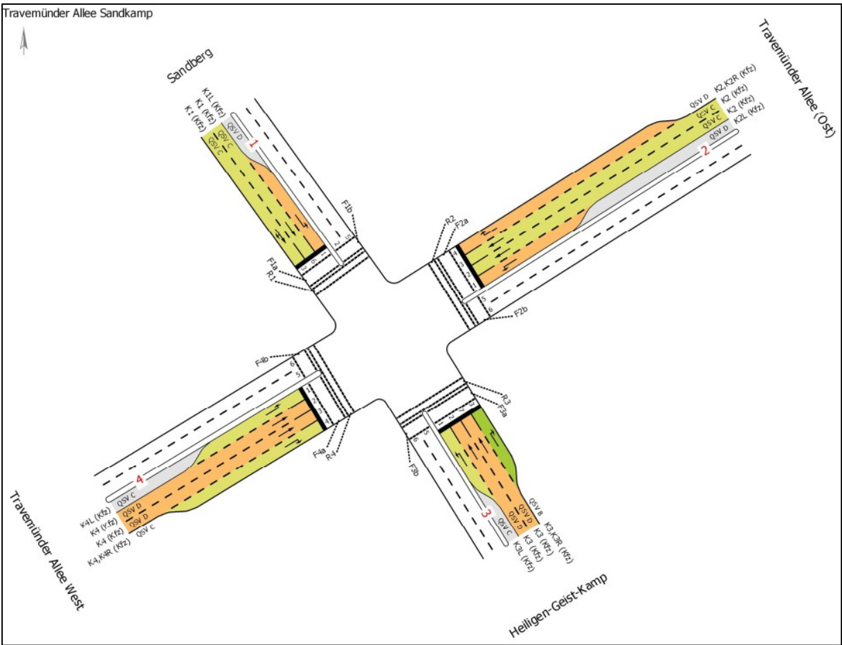
Abbildung 3: Skizze Verkehrsqualitätsstufen Planung (Prognose 2035)
