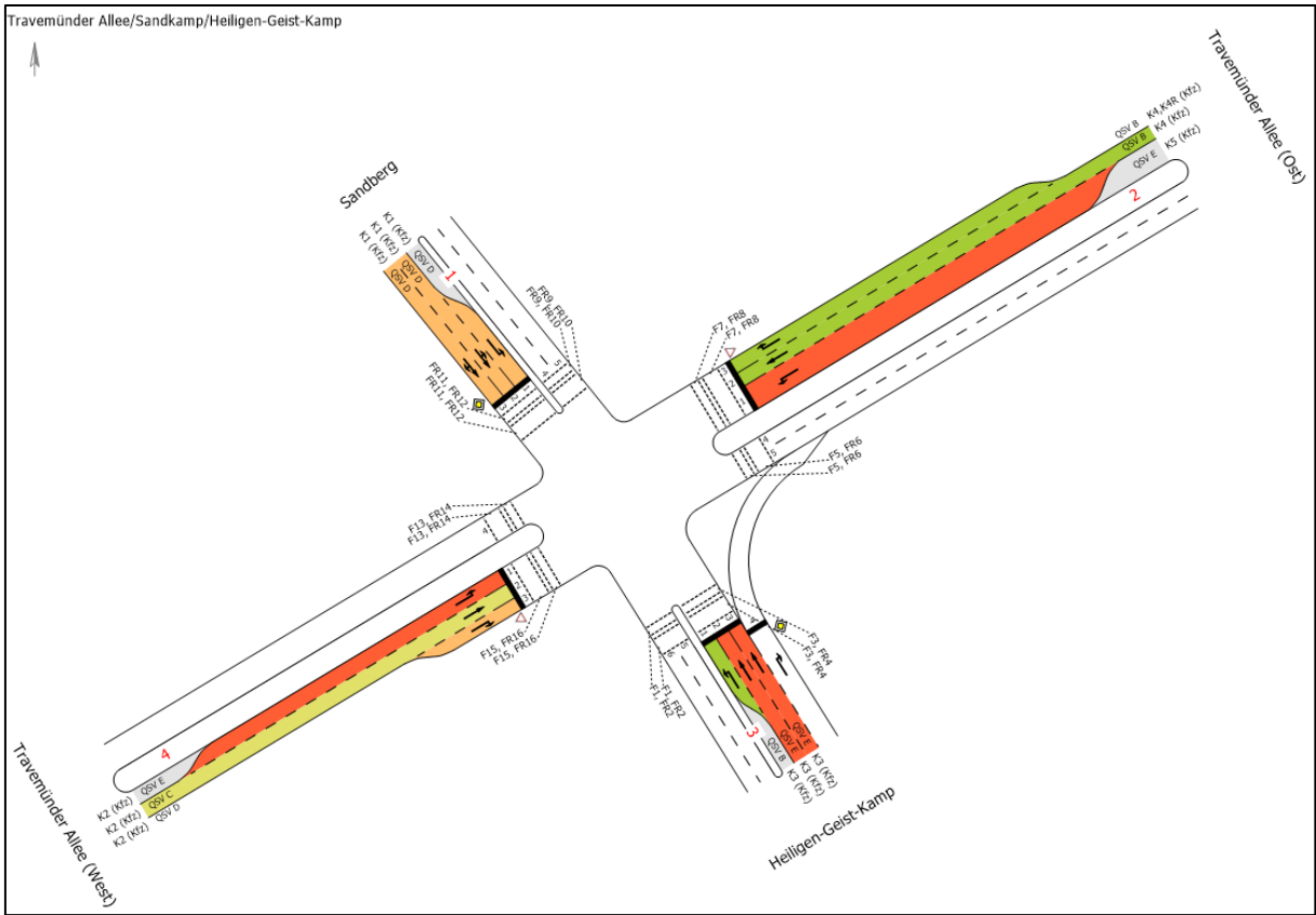
Abbildung 2: Skizze Verkehrsqualitätsstufen Bestand (Prognose 2035)
