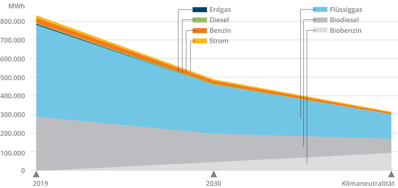
Abbildung 17: Entwicklung der Energiebedarfe im Sektor Mobilität im Minderungspfad Treibhausgasneutralität 2040 (energielenker 2021)
