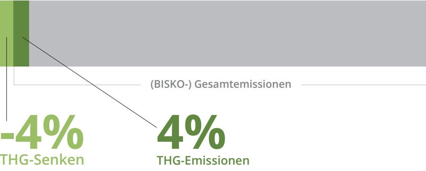
Abbildung 29: Übersicht der Treibhausgasemissionen und -senken in Lübeck
