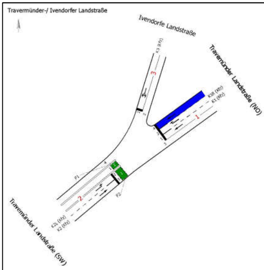
KP01 – schematische Knotenpunktdarstellung 2035 (P0)
