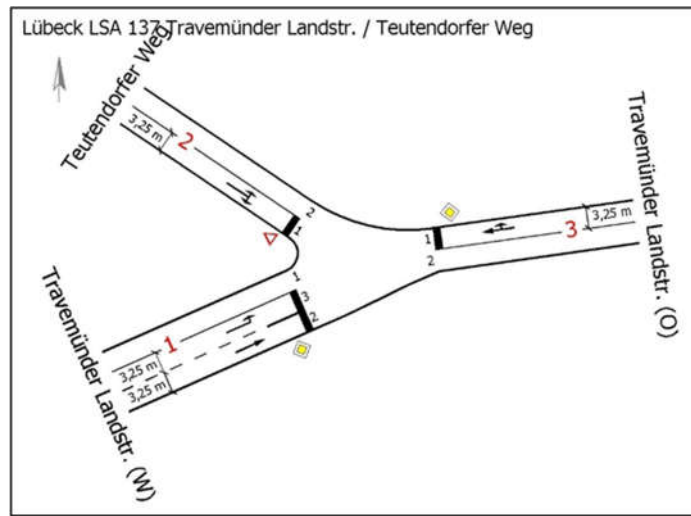
KP07 – schematische Knotenpunktdarstellung 2035 (P2)
