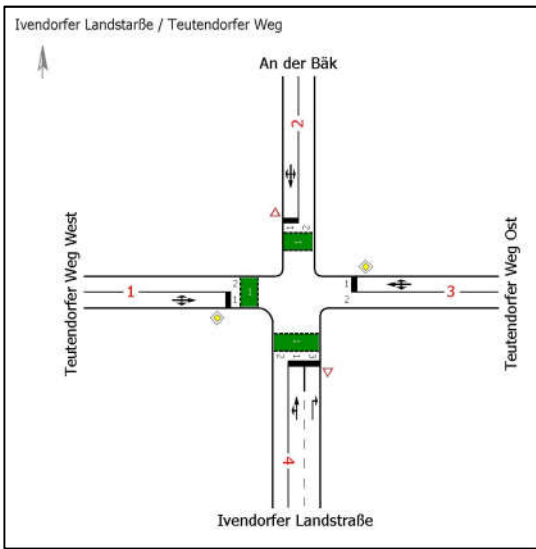
KP08 – schematische Knotenpunktdarstellung 2035 (P5)
