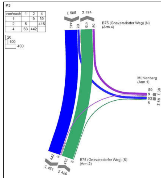
KP04 – Knotenstrombelastung Spitzenstunde 2035 (P3)
