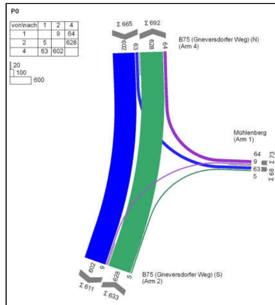
KP04 – Knotenstrombelastung Spitzenstunde 2035 (P0)
