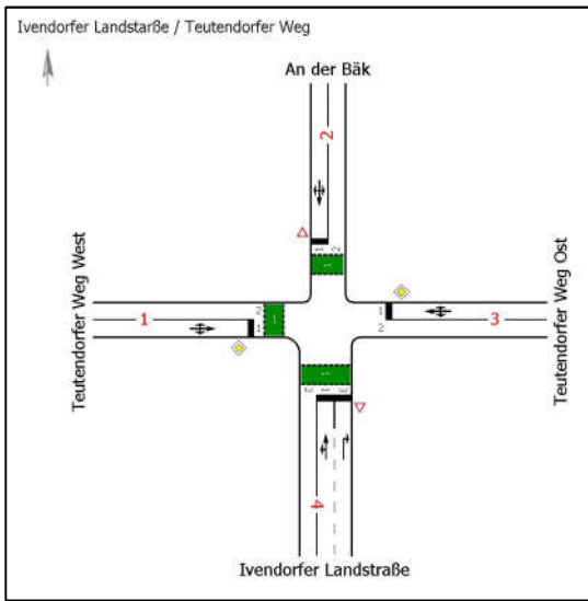
KP08 – schematische Knotenpunktdarstellung 2035 (P2)
