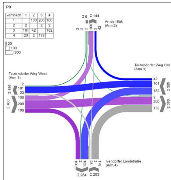
KP08 – Knotenstrombelastung Spitzenstunde 2035 (P0)
