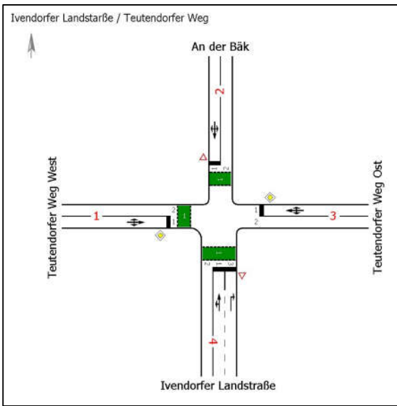
KP08 – schematische Knotenpunktdarstellung 2035 (P0)
