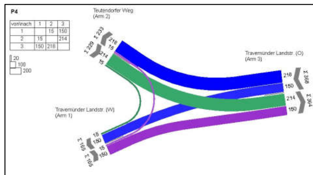
KP07 – Knotenstrombelastung Spitzenstunde 2035 (P4)
