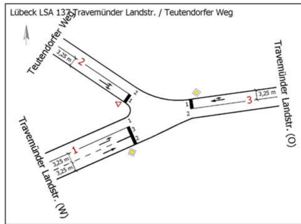
KP07 – schematische Knotenpunktdarstellung 2035 (P4)
