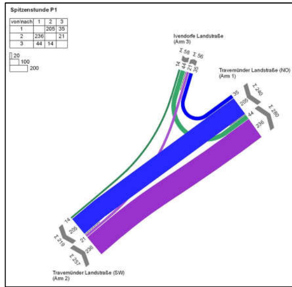
KP01 – Knotenstrombelastung Spitzenstunde 2035 (P1)
