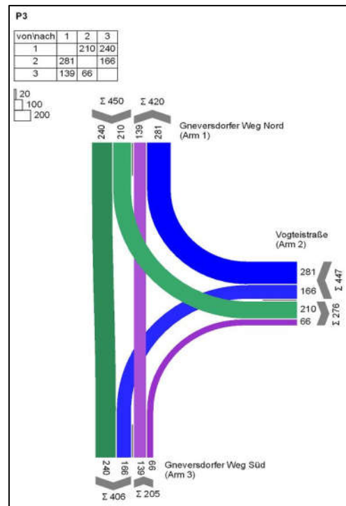
KP05 – Knotenstrombelastung Spätspitze 2035 (P3)
