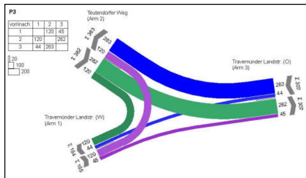
KP07 – Knotenstrombelastung Spitzenstunde 2035 (P3)
