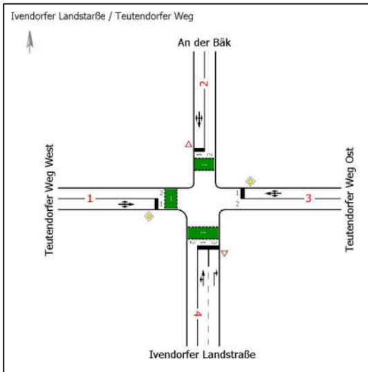
KP08 – schematische Knotenpunktdarstellung Analyse 2021
