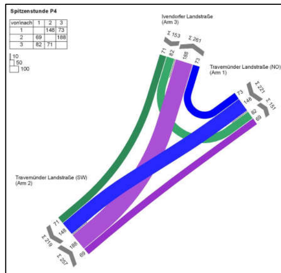
KP01 – Knotenstrombelastung Spitzenstunde 2035 (P4)
