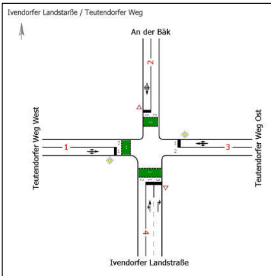
KP08 – schematische Knotenpunktdarstellung 2035 (P4)
