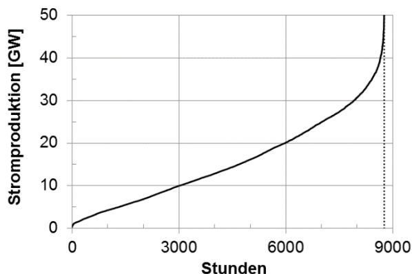
Abbildung 25: Stromproduktion PV + Wind in aufsteigend geordneten Stundenwerten für das Jahr 2017, Daten aus [ISE4]
