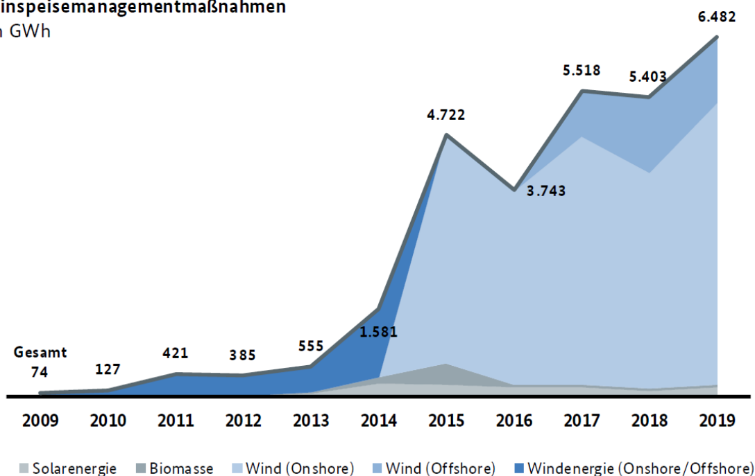
Abbildung 22: Abgeregelter elektrische Energie [BNA]
