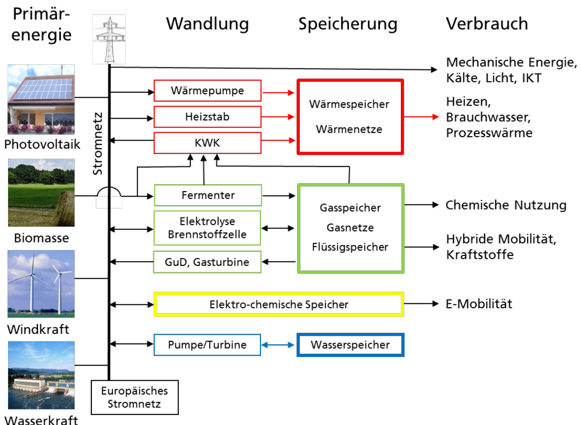
Abbildung 59: Vereinfachte schematische Darstellung eines Erneuerbaren Energiesystems mit den wichtigsten stromnetzgebundenen Bausteinen der Gewinnung, Wandlung, Speicherung und des Verbrauchs
