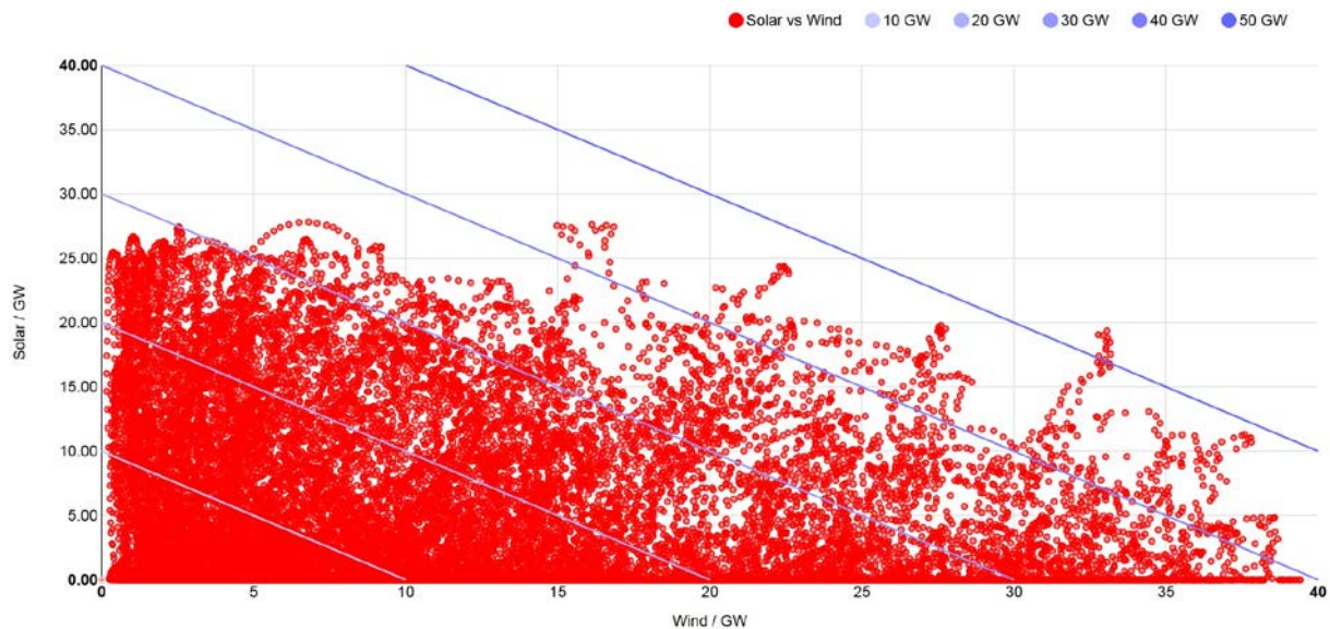
Abbildung 24: Mittlere Leistung für die Einspeisung von Sonnen- und Windstrom im Jahr 2017, 15-Minuten-Werte [ISE4]
