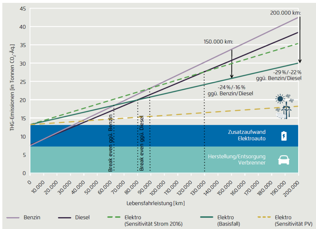
Abbildung 53: Treibhausgasemissionen von heutigen Fahrzeugen der Kompaktklasse in Abhängigkeit von der Fahrleistung [AGORA2]
