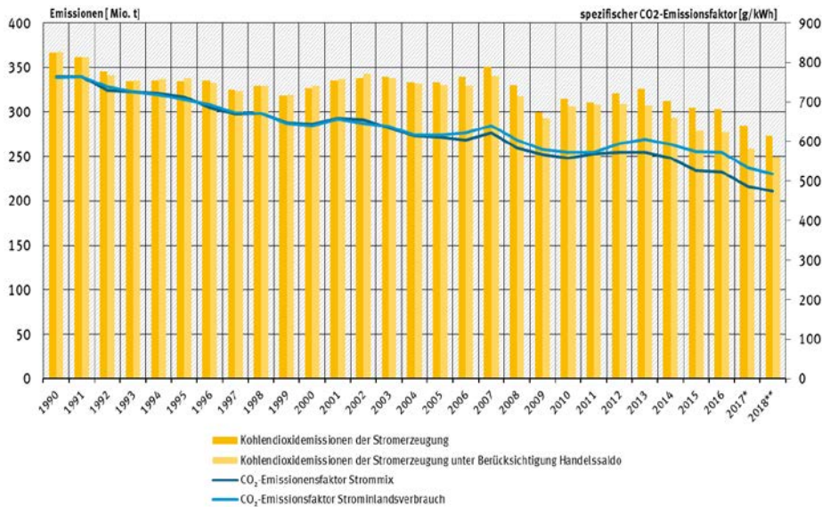
Abbildung 39: Spezifische und absolute CO 2 -Emissionen der Stromerzeugung in Deutschland [UBA6]
