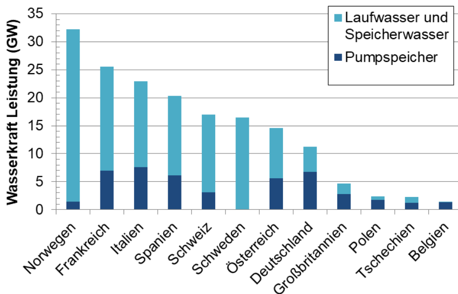
Abbildung 58: Installierte Leistung von Wasserkraftwerken in benachbarten Ländern, Zahlen aus [IHA]
