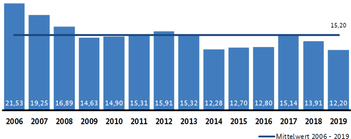
Abbildung 28: System Average Interruption Duration Index (SAIDI) für in Minuten/Jahr [BNA]
