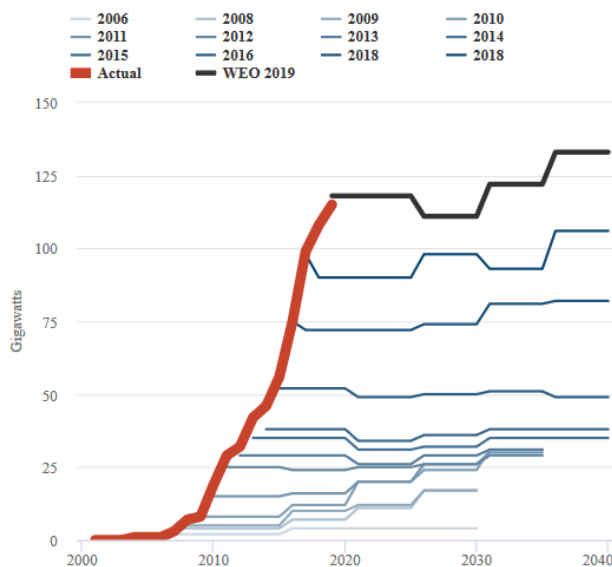
Abbildung 49: IEA-Prognosen seit 2006 und tatsächliche Entwicklung des globalen jährlichen PV-Zubaus [Carb]
