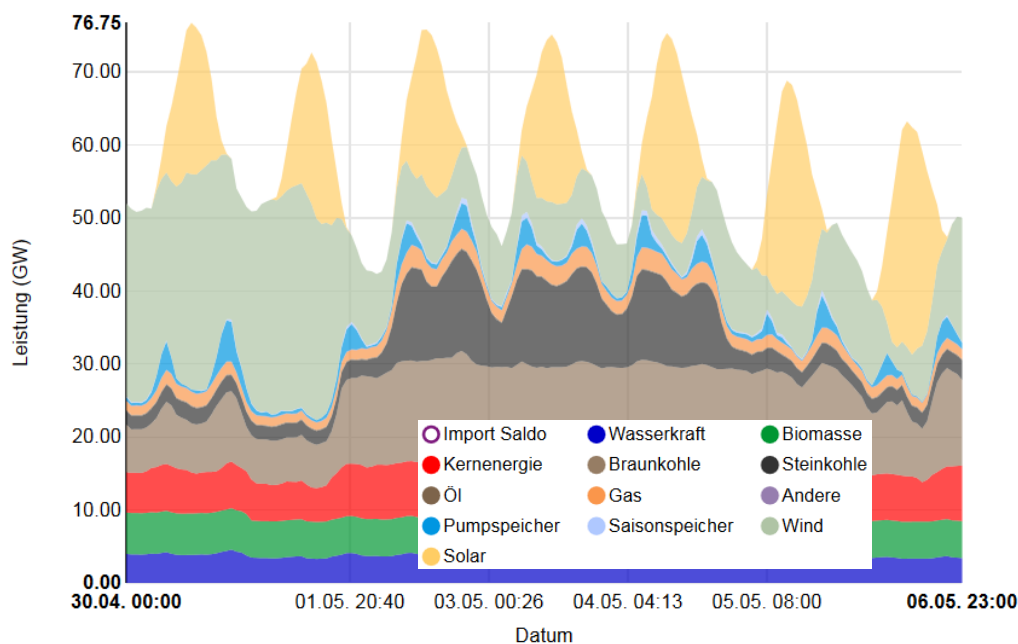
Abbildung 27: Beispiel für den Verlauf von Börsenstrompreisen, konventioneller und regenerativer Stromerzeugung der 18. Kalenderwoche im Mai 2018 [ISE4]
