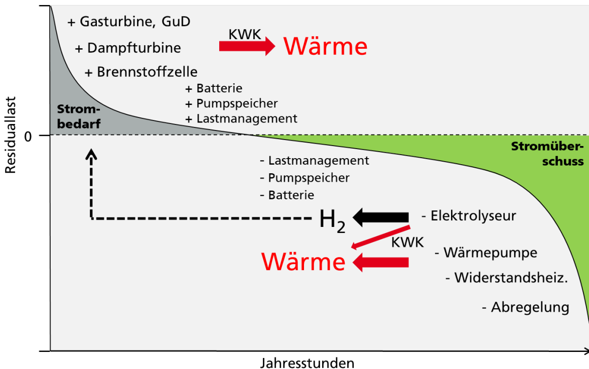
Abbildung 47: Schematische Darstellung einer Residuallastkurve für Deutschland bei Stromversorgung mit 100% EE, mit Erzeugern (+) und Lasten (-)
