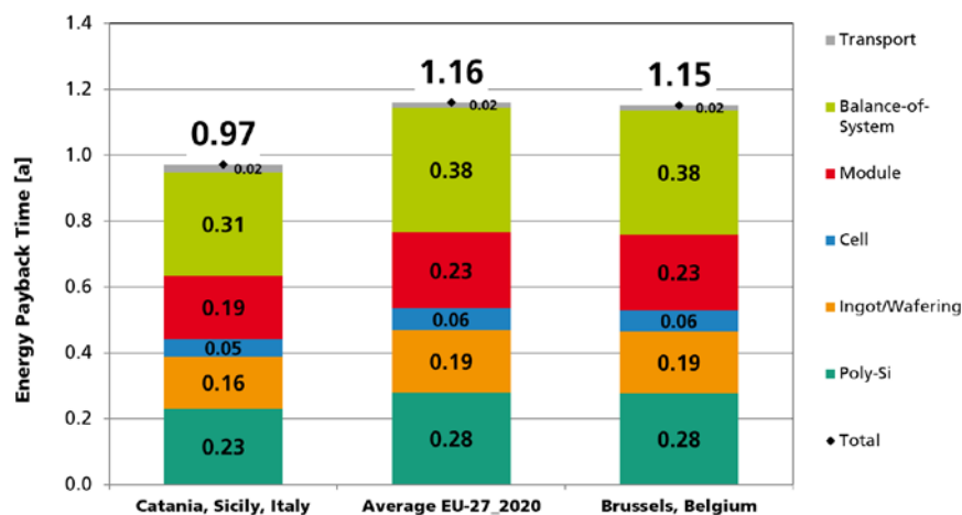
Abbildung 29: Berechnete Energierücklaufzeiten von PV-Kraftwerken für europäische Produktions- und Betriebsstandorte [ISE10], Daten: Lorenz Friedrich
