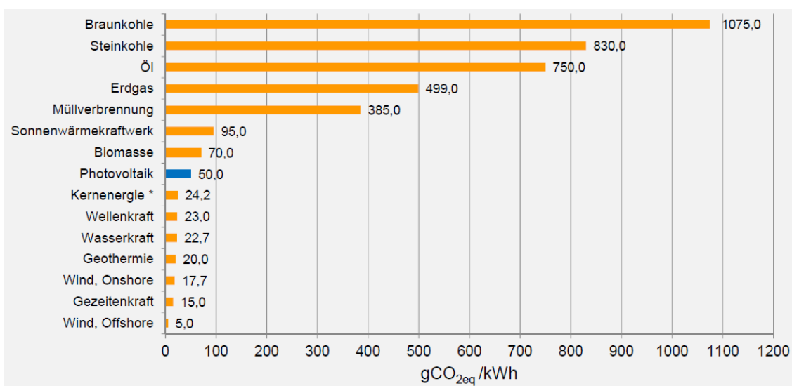
Abbildung 38: Durchschnittliche CO 2 -Äquivalent Emissionen verschiedener Stromerzeugungstechnologien [EnAg]
