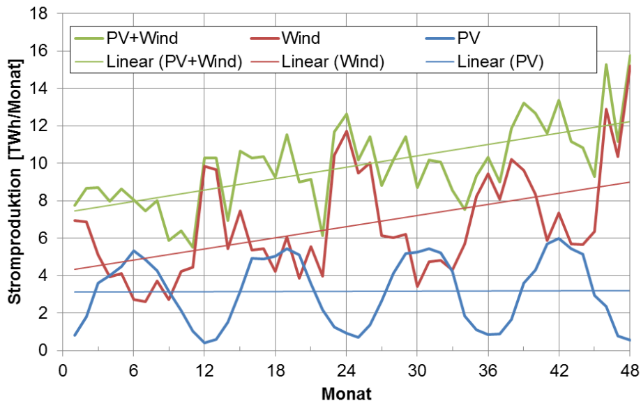
Abbildung 26: Monatliche PV- und Windstromproduktion der Jahre 2014-2017 [ISE4]
