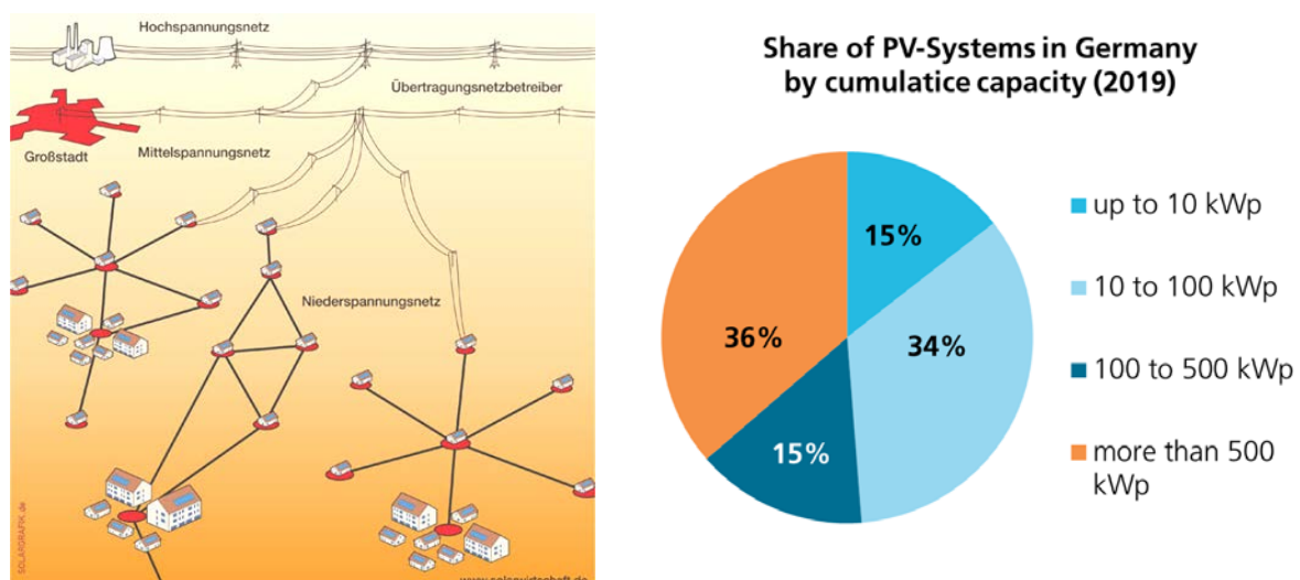
Abbildung 21: Links: Einspeisung von PV-Strom [BSW], Rechts: Verteilung der installierten PV-Leistung nach Anlagengröße [ISE10]
