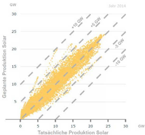
Abbildung 23: Stündliche tatsächliche und geplante Stromproduktion im Jahr 2014 [ISE4]
