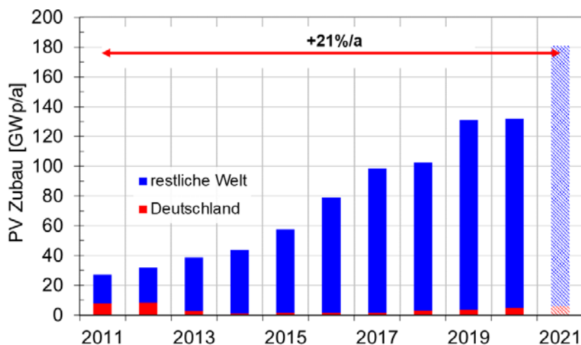
Abbildung 41: Entwicklung des jährlichen PV-Zubaus für Deutschland und die restliche Welt, Zahlen von EPIA, IHS, Solar Power Europe, mit Prognose für 2021.
