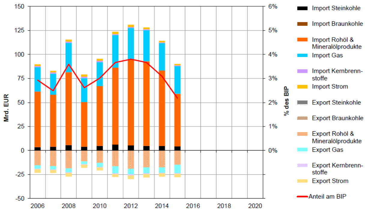
Abbildung 44: Entwicklung der Kosten für die Bereitstellung der Primärenergie in Deutschland [ÖKO3]
