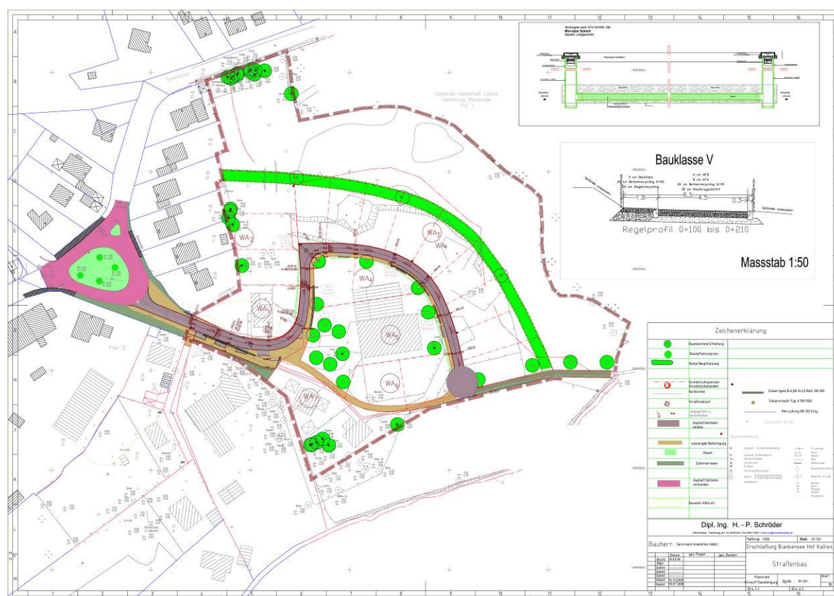
Abb. 5: unverbindliche Skizze Erschließung B-Plan 10.04.00 (Stand: 10.07.2008)
