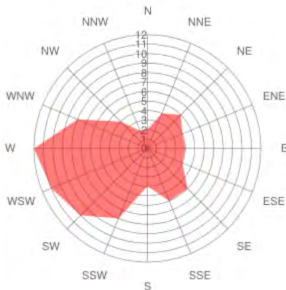
Abb. 5-1: Angaben zur Windrichtungsverteilung und zur Häufigkeit der Windgeschwindigkeiten
