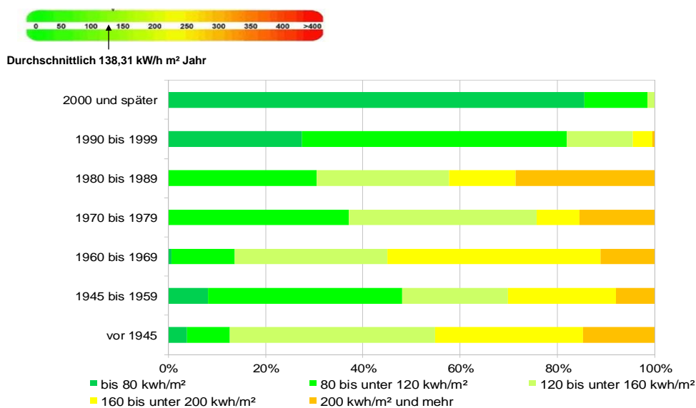
Abb. 8: Energieverbrauch nach Baualter (Datenabfrage Wohnungswirtschaft)
